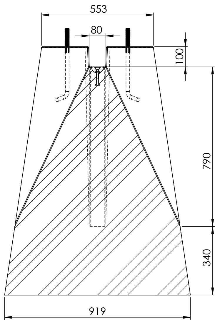
COUPE A-A ECHELLE 1 : 11
