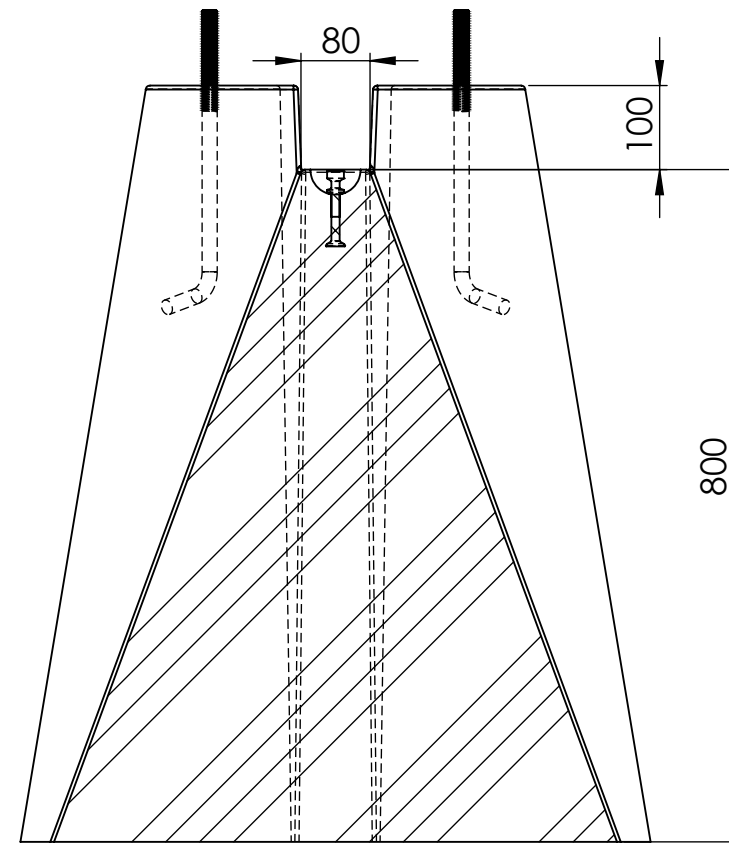
COUPE A-A ECHELLE 1 : 9
